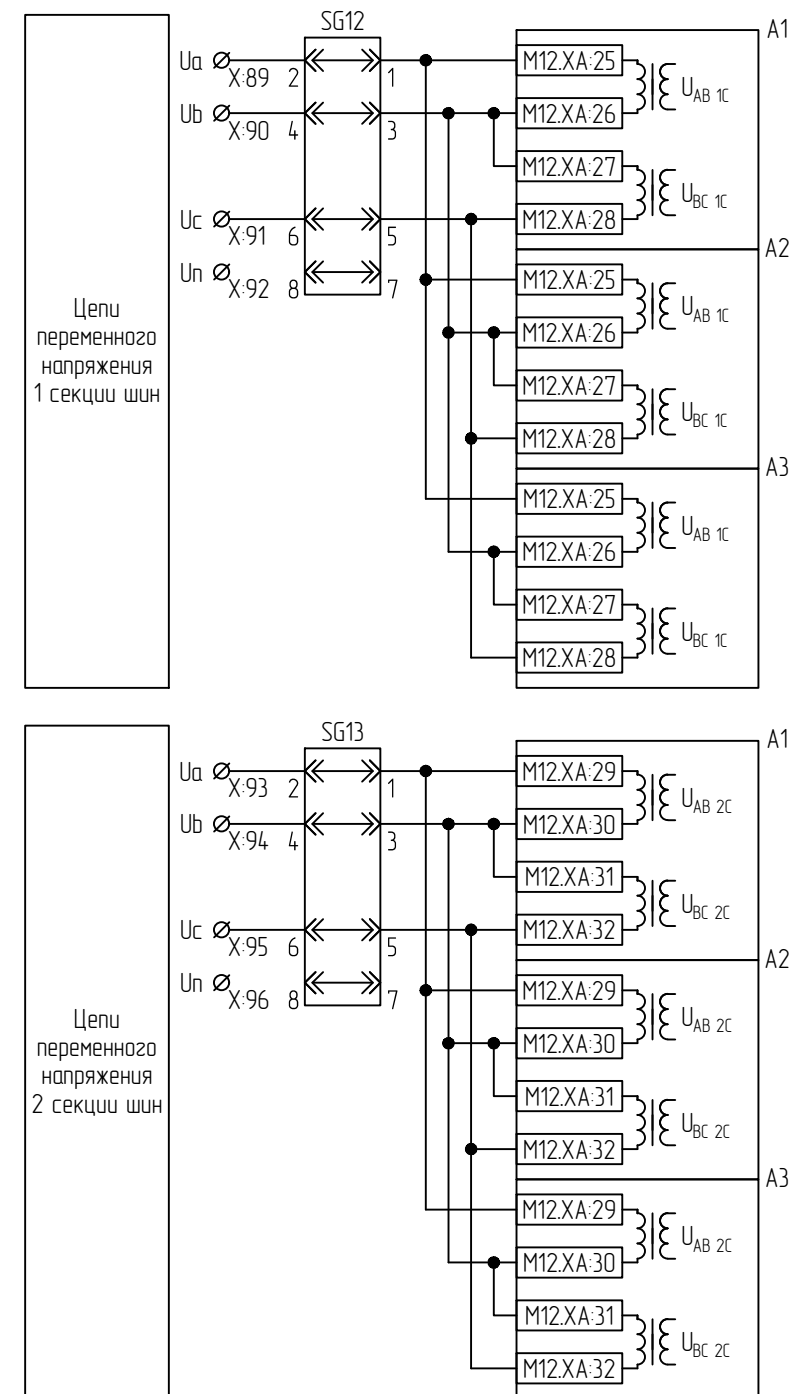
Цепи переменного напряжения
