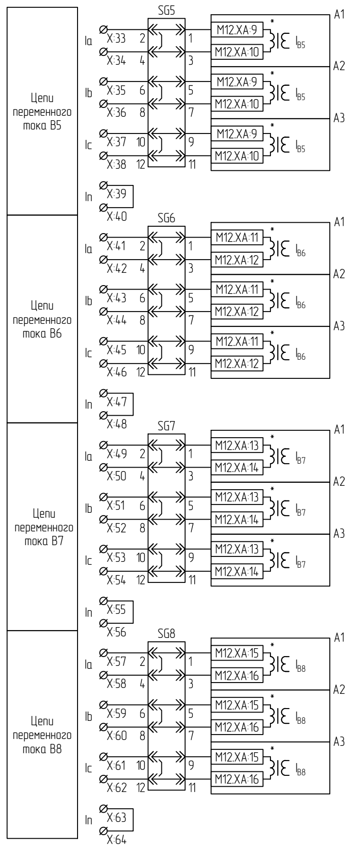
Цепи переменного тока
